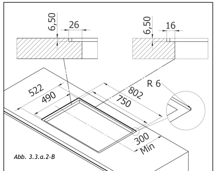
Abb. 3.3.a.2-B -> 80 cm Platte.
