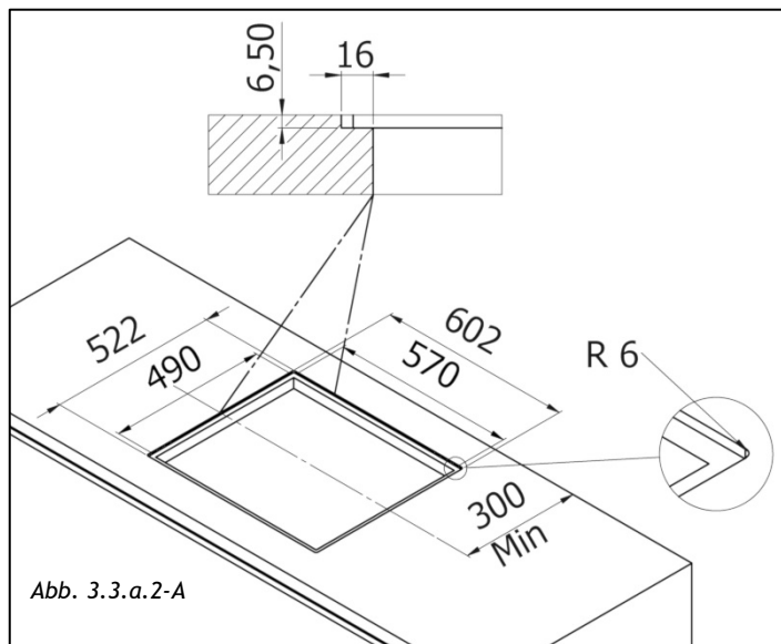
Abb. 3.3.a.2-A -> 60 cm Platte.
