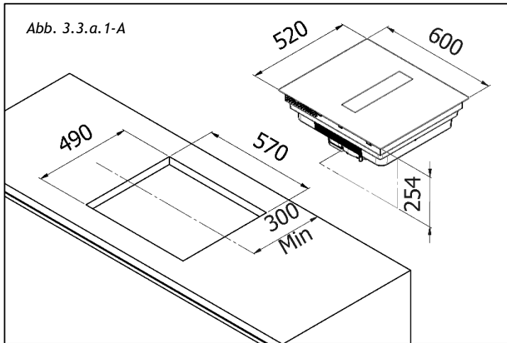
Abb. 3.3.a.1-A -> 60 cm Platte.
